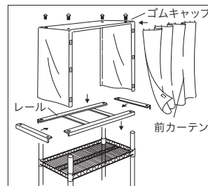
〈取り付け図〉
