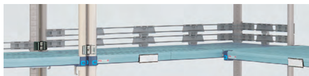
サイドレージ2段の場合
