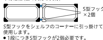
S型フック M9995
