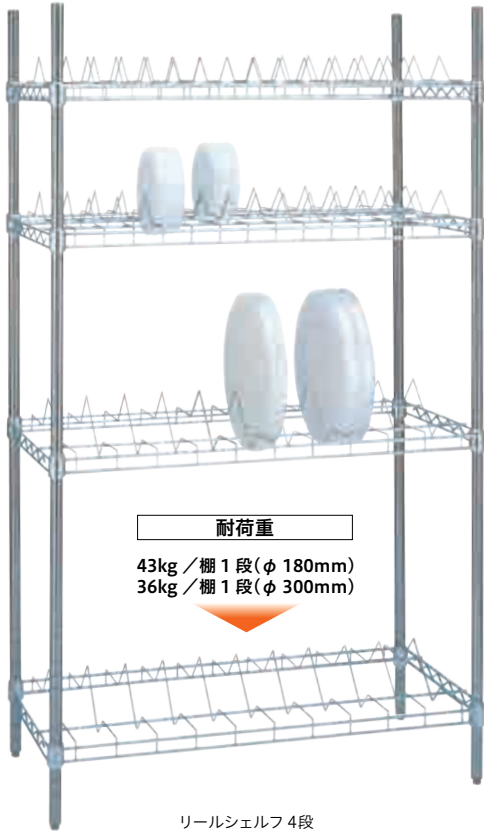
リールシェルフ 4段 外寸：W910×D460×H1587mm
